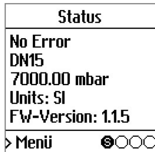
Fig. 19 Status display
