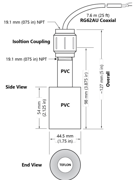
PZ32T sensor
