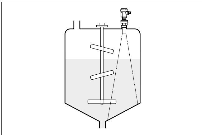
Fig. 12: Agitators
