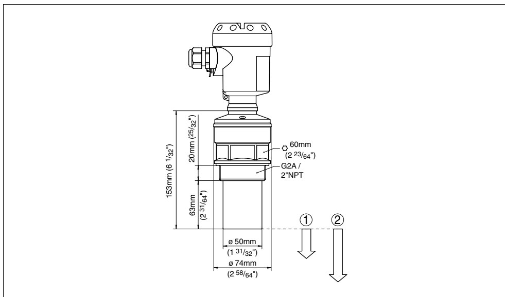
Fig. 28: OPTISOUND 3020 C
