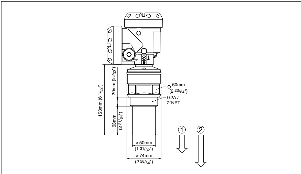
Fig. 23: OPTISOUND 3020 C
