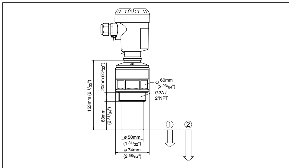
Fig. 26: OPTISOUND 3020 C
