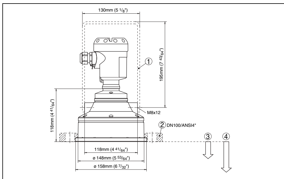
Fig. 27: OPTISOUND 3030 C
