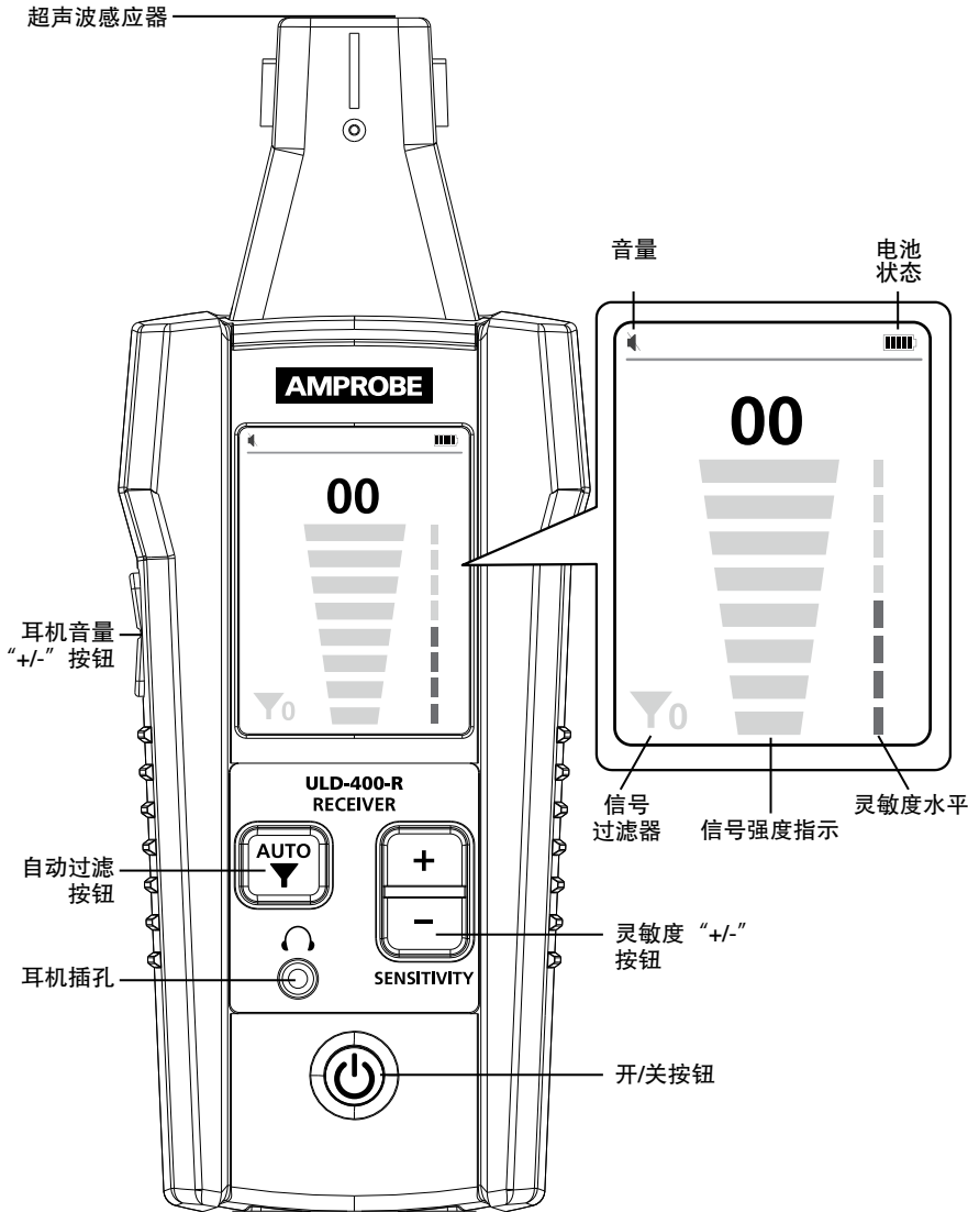
图3.2： ULD-400-R接收器
