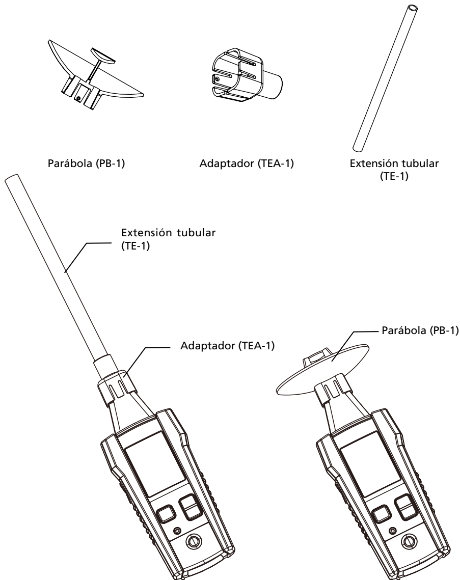
Figura 3.4: Accesorios ULD-400
