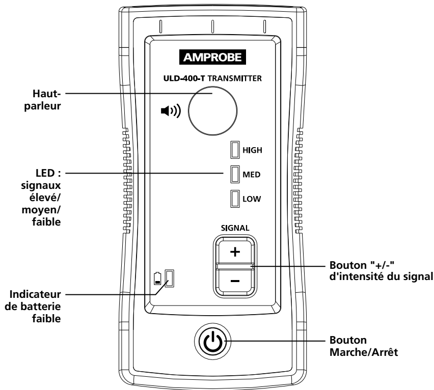
Figure 3.3 : Émetteur ULD-400-T
