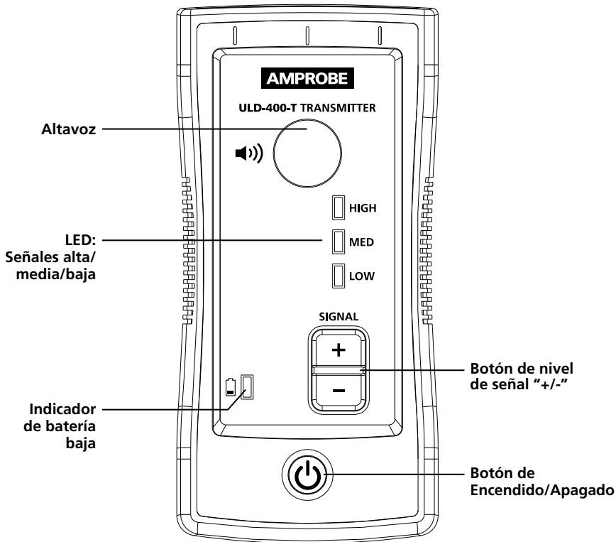
Figura 3.3: Transmisor ULD-400-T
