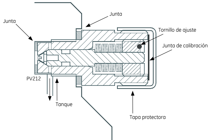
PRV212 Esquema
